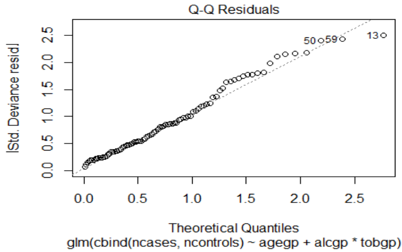
Figure 2: The Q-Q (quantile-quantile) plot
